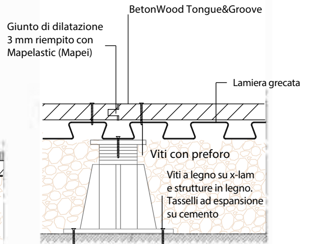
Giunti di dilatazione della soluzione con BetonWood Tongue&Groove
