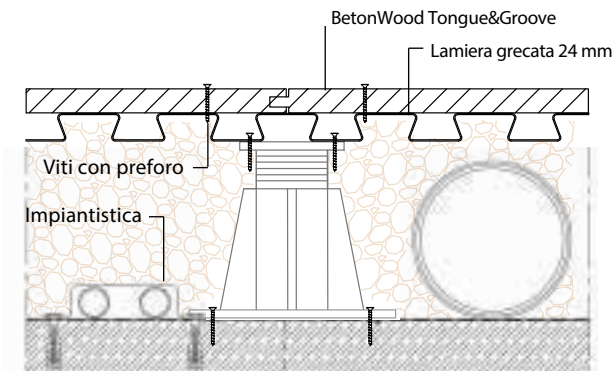
Utilizzo dell'intercapedine per passaggio impianti
